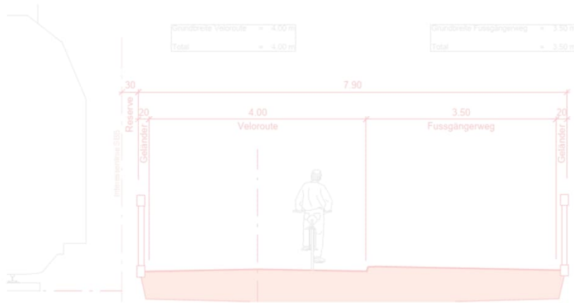
Abbildung 21: Normalprofil Brücke. Eigene Darstellung.
